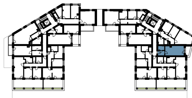
SCHÉMATICKÝ PŮDORYS
